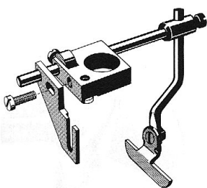
Edge ruler 13,1 mm
