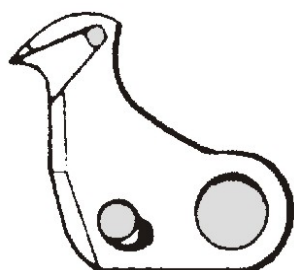
Juki Messer
